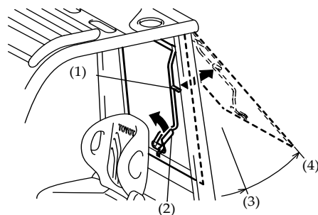
(1) Levier d'assistance (2) Levier de blocage (3) Mode de ventilation (4) Mode de maintenance
