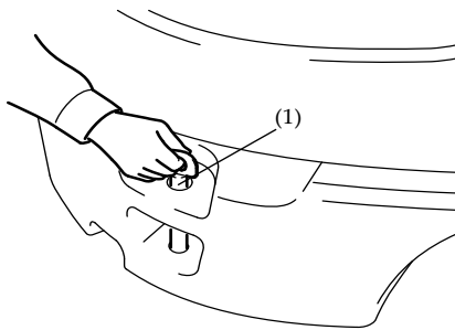
(1) Barre d'attelage
