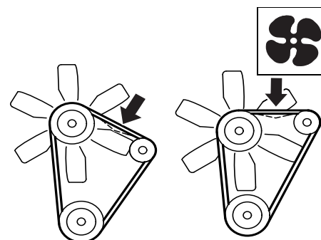
Moteur 4Y
