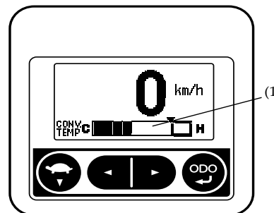
(1) Jauge de température de l'huile du convertisseur de couple
