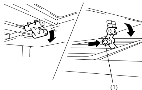
(1) Bouton de déverrouillage
