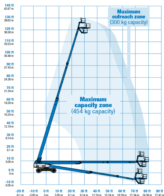
Courbe de travail SX-125 XC
