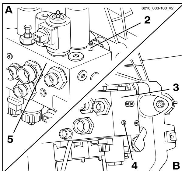
A Version joystick 4Plus et version à mini-levier : B Version multi-leviers
