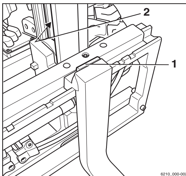
Bras de fourche et rails de roulement
