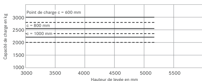
RX 60-30/600 Téléscoptique/NiHo
