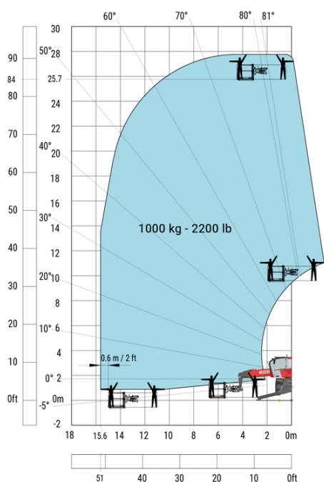
Machine sur stabilisateurs abaissés avec nacelle 3D négatif Machine sur stabilisateurs abaissés avec potence-treuil extensible (Métrique)
