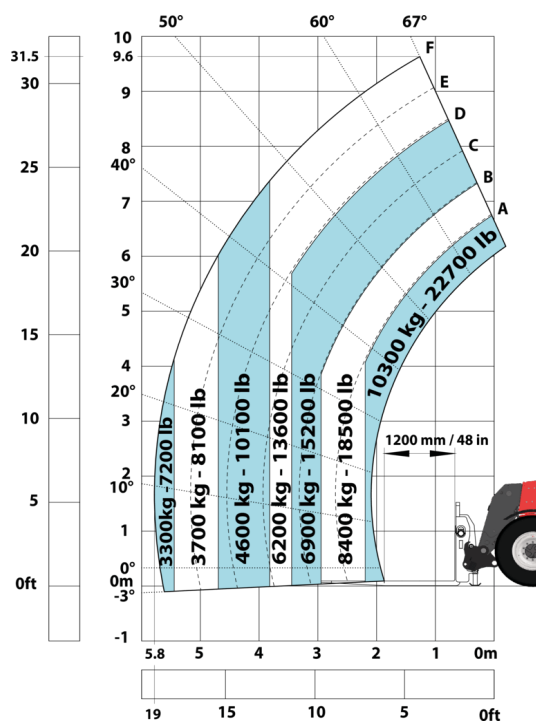
Machine sur pneus avec fourches LC 1200 mm Mètric
