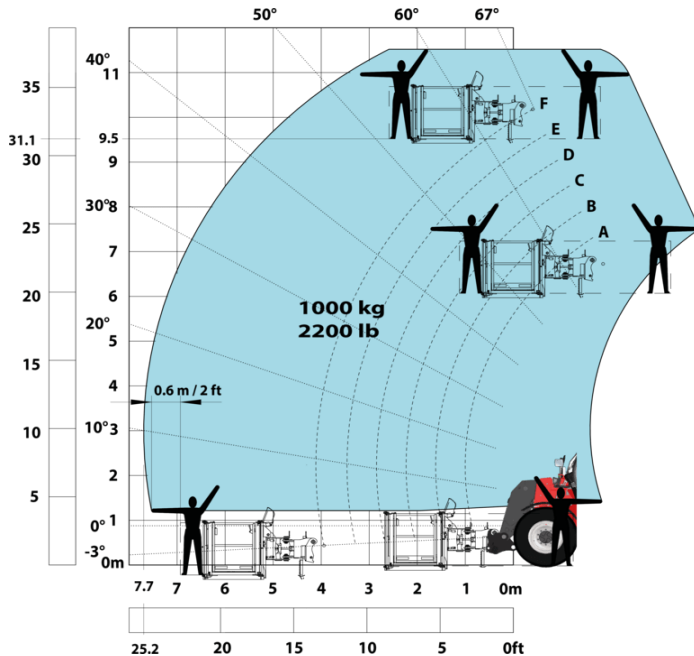
Machine sur pneus avec nacelle Mètric
