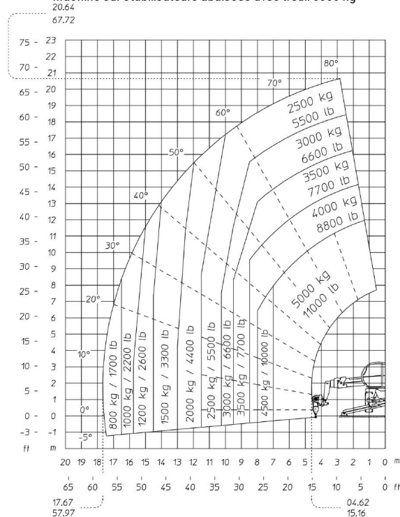
Machine sur stabilisateurs abaissés avec treuil 5000 kg
