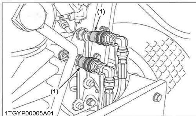
(1) Sortie hydraulique (si équipé)
