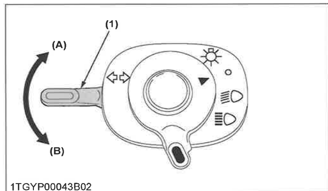
1TGYP00043B02 (1) Commande de clignotants de direction (A) « CLIGNOTANT DROIT » (B) « CLIGNOTANT GAUCHE »
