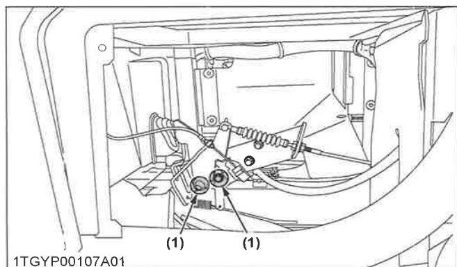
(1) Pédale de blocage du différentiel (de type pulvérisation de graisse)
