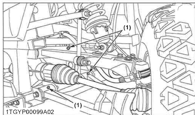
(1) A-ARM avant (point de graissage)
