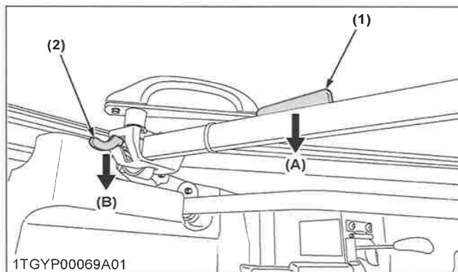
1TGY00069A01 (1) Poignée de porte (A) « APPUYER » (2) Poignée intérieure (B) « TIRER »
