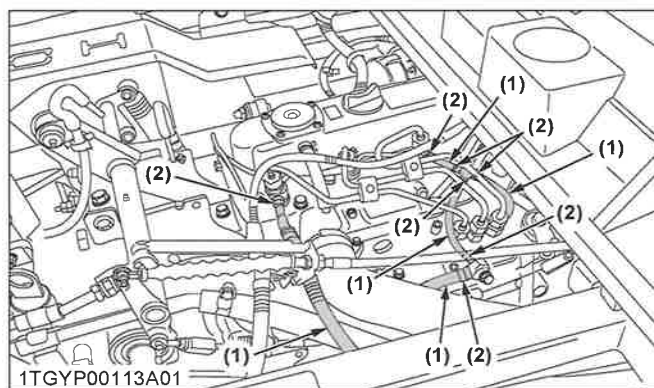
(1) Tuyau d'alimentation en carburant (2) Collier de tuyau
