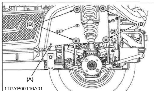
(A) Garde-boue
