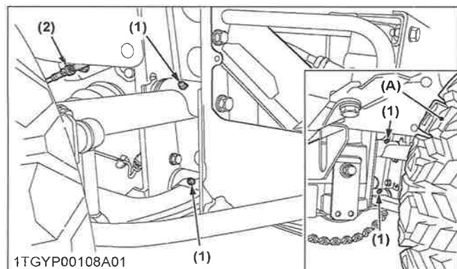
(1) A-ARM arrière (point de graissage) (A) Pneu arrière gauche (2) Liaison de frein de stationnement (de type pulvérisation de graisse)
