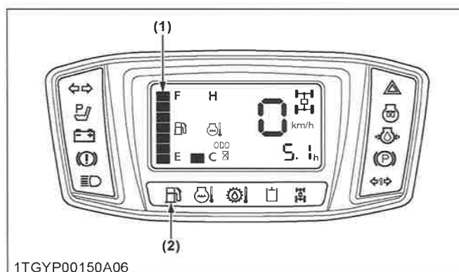
(1) Jauge à carburant
