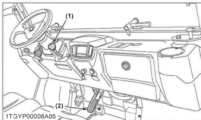
(1) Levier de changement de gamme (2) Pédale de commande de vitesse
