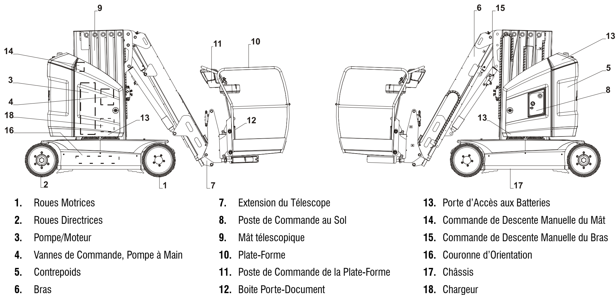
Figure 3-3. Nomenclature - Localisation des Commandes de la Machine
