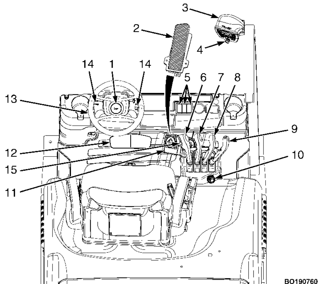
Figure 7. Commandes du cariste - Commandes hydrauliques manuelles
