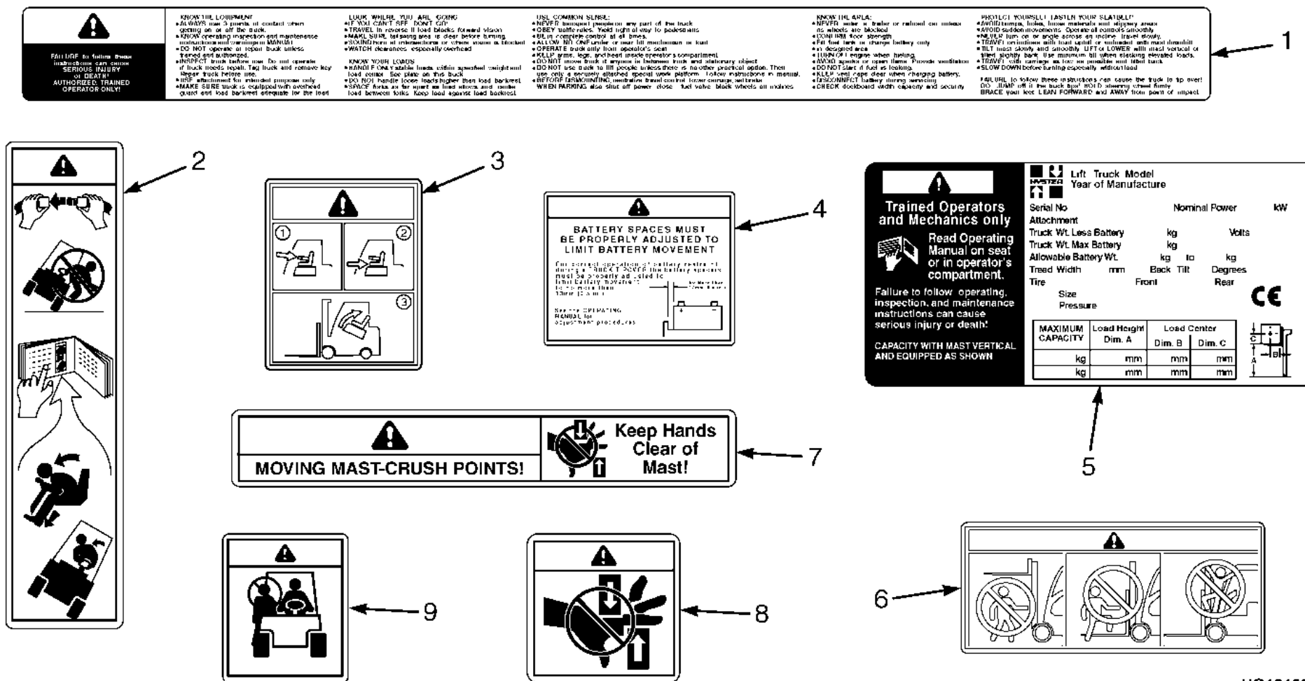
Figure 6. Étiquettes d'avertissement et de sécurité
