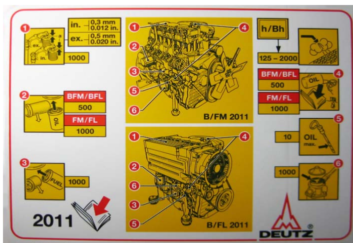
Autocollant des consignes d'entretien pour le moteur diesel
