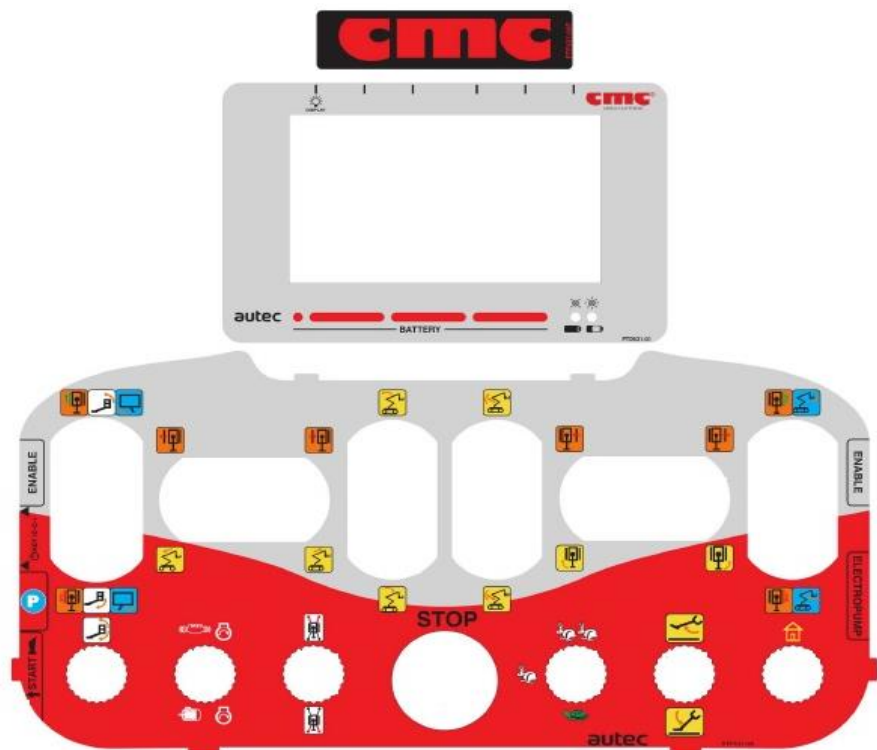
Figure 68 : radiocommande AUTEC.
